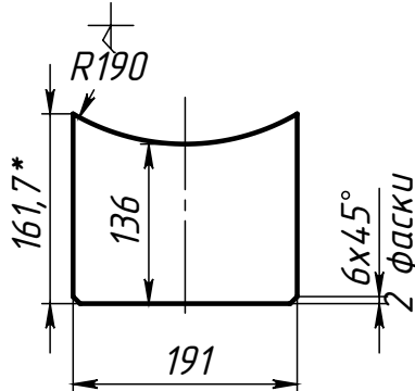
Поз.3 (Ребро среднее)
