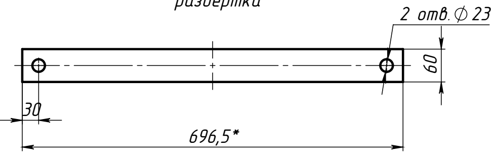
Поз.4 (Полухомут) развертка
