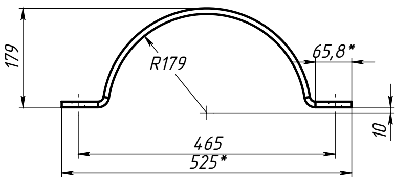
Поз.4 (Полухомут)
